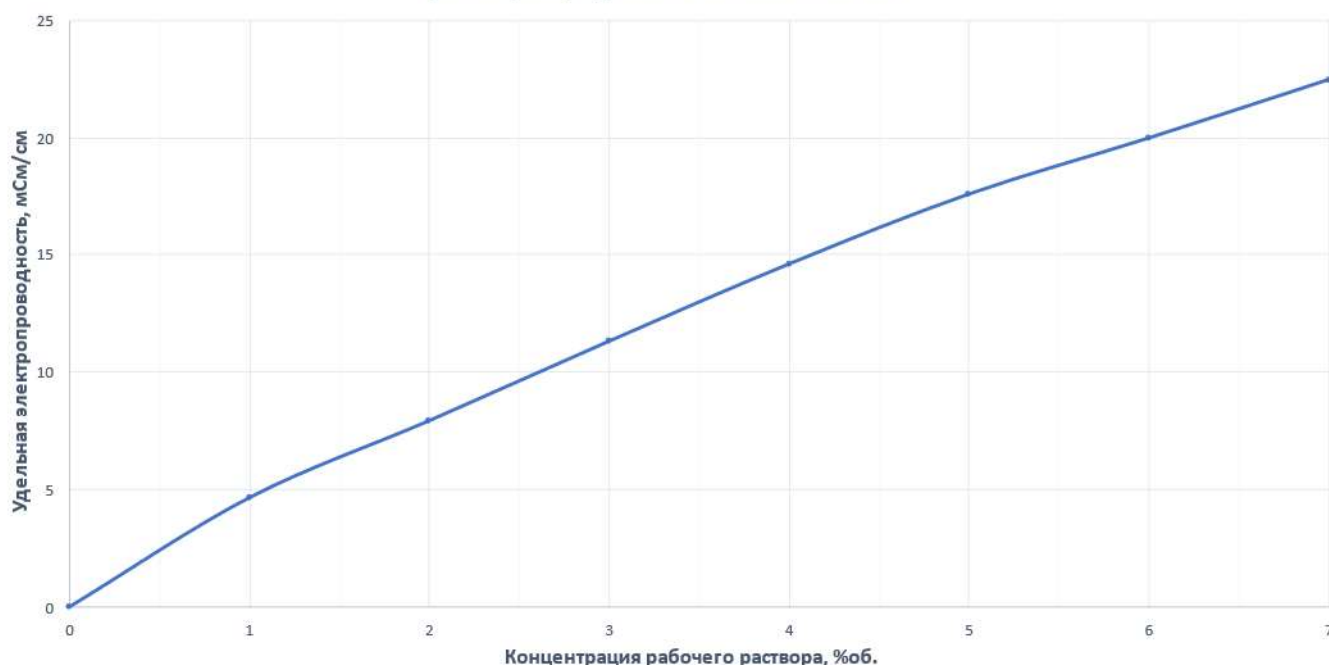
График зависимости удельной электропроводности от концентрации рабочего раствора средства Transfoam Chlor Alu
